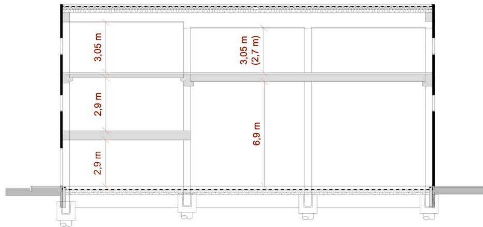
Řez příčný
